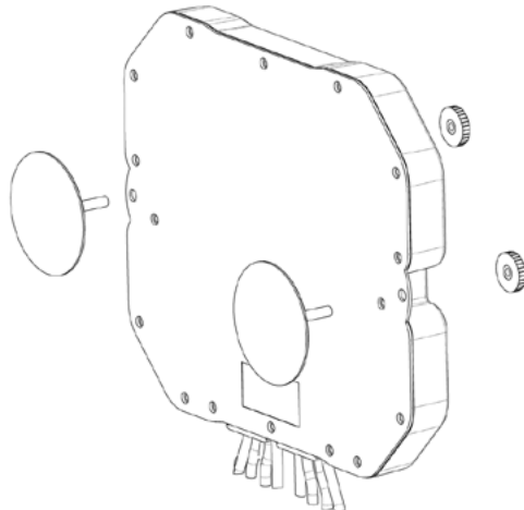
fig 7. Fixation à ventouse où le GPS n'est pas utilisé ou l'antenne est montée horizontalement
