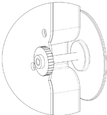
fig 10. La tuerca debe estar al ras con la cabeza de la rosca integrada para permitir un agarre adecuado en la orientación frontal
