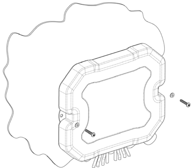
fig 5. Fixation verticale à l'aide de vis
